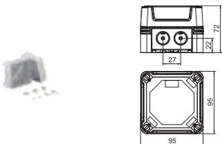
Abmessungen
